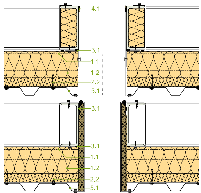
Seitliche Toranschlüsse
