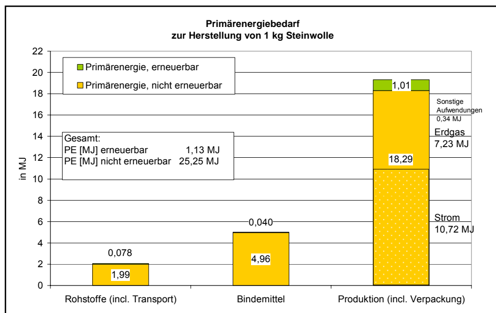
Abbildung 2: Primärenergiebedarf zur Herstellung von 1 kg Steinwolle
